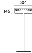
POFE50 (1) POFD50 (2) H * L 400 D 305
