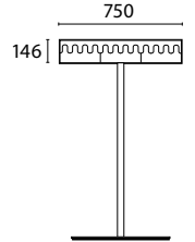
POFE75 (1) POFD75 (2) H * L 610 D 305
