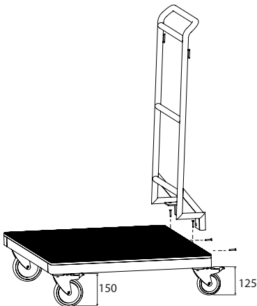
Handtaget på långsida, plats för 7 bord. Handle long side, 7 tables.
