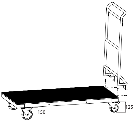
Handtaget på kortsida, plats för 13 bord. Handle short side, 13 tables.
