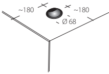
TKB5 Kabelgenomföring. Cable slot.
