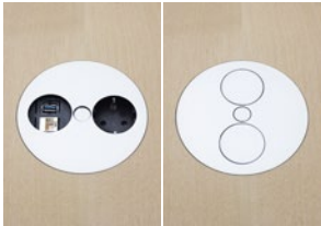
TKB10 Ø 115 mm Ett eluttag. Två USB laddare. Lock borstat rostfritt stål. Två meter kabel. Gäller för SE, NO, DK, FIN, DE, NL. One electrical. Two USB charging. Mattchrome lid incl. Two meters cables. For SE, NO, DK, FIN, DE, NL.
