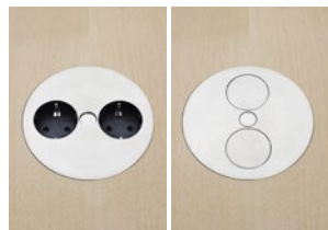
TKB7 Ø 115 mm Två eluttag. Lock borstat rostfritt stål. Två meter kabel. Gäller för SE, NO, DK, FIN, DE, NL. Two electrical. Mattchrome lid. Two meters cable. For SE, NO, DK, FIN, DE, NL.
