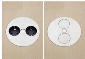
TKB7 Ø 115 mm Twist. Två eluttag. Lock borstat rostfritt stål. Två meter kabel. Gäller för SE, NO, DK, FIN, DE, NL. Twist. Two electrical. Brushed stainless lid. Two meters cable. For SE, NO, DK, FIN, DE, NL.
