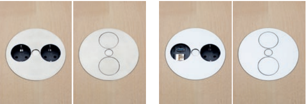
TKB7 Ø 115 mm Två eluttag. Lock borstat rostfritt stål. Två meter kabel. Gäller för SE, NO, DK, FIN, DE, NL. Two electrical. Brushed stainless lid. Two meters cable. For SE, NO, DK, FIN, DE, NL.
