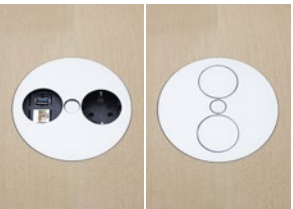
TKB10R Ø 115 mm Twist. Ett eluttag. Två USB A laddare. Lock borstat rostfritt stål. Två meter kabel. Placering ovanför träbalk. Gäller för SE, NO, DK, FIN, DE, NL. Twist. One electrical. Two USB A charging. Brushed stainless lid. Two meters cables. Placed above wooden beam. For SE, NO, DK, FIN, DE, NL.
