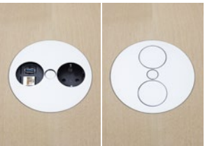
TKB10R Ø 115 mm Ett eluttag, Två USB A laddare. Lock borstat rostfritt stål. Två meter kabel. Placering ovanför träbalk. Gäller för SE, NO, DK, FIN, DE, NL. One electrical. Two USB A charging. Brushed stainless lid. Two meters cables. Placed above wooden beam. For SE, NO, DK, FIN, DE, NL.
