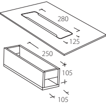
TKB4 Kabelgenomföring med elbrunn. Lösa lock. Endast till rektangulär skiva. Cable slot with box. For socket and leads. Loose covers. Only rectangular top.
