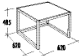
269-1 massiv skiva 269-2 glas
